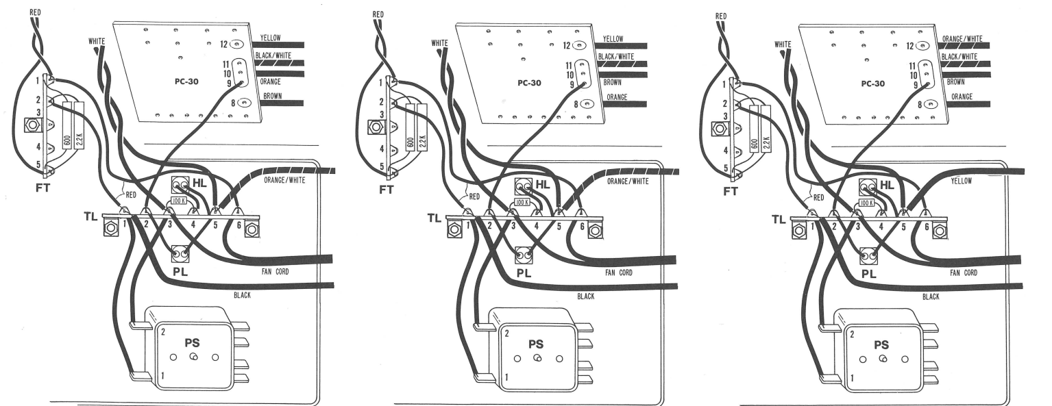
240 VAC
